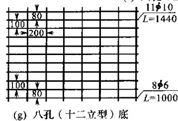
图 7.3.6 管道基础进入人(手)孔处配筋
