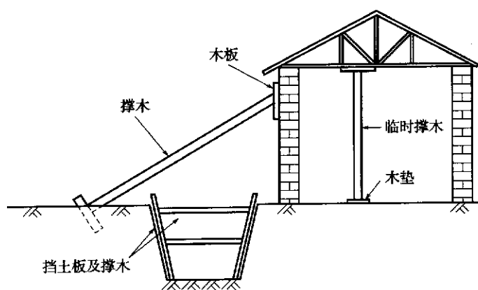
图 1 房屋支撑
