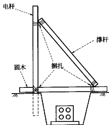
图 2 电杆支撑
