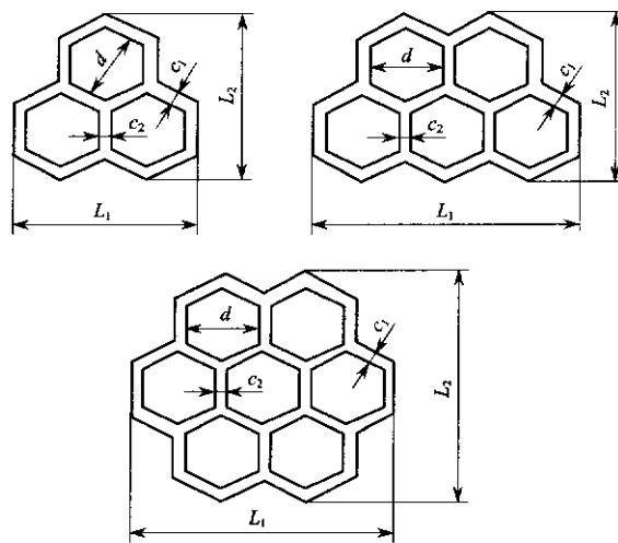
图 B.0.2-2 蜂窝管截面
