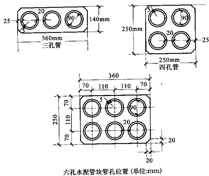
图 B.0.1 水泥管块规格示意
