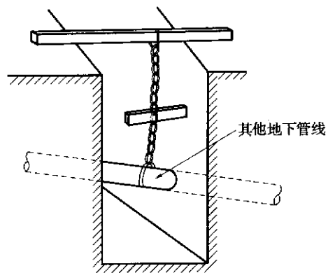
图 3 其他管线与管沟交越保护
