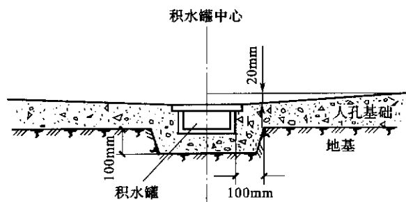
图 6.2.4 人(手)孔、通道基础断面
