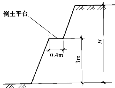
图 4.1.5 增设倒土平台
